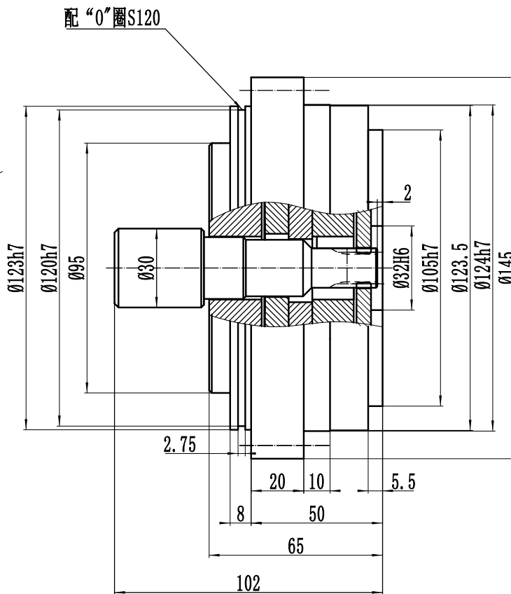
标准“B”型输入轴
