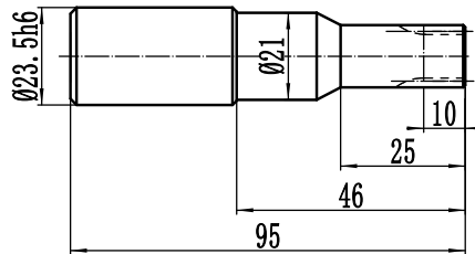
标准“A”型输入轴
